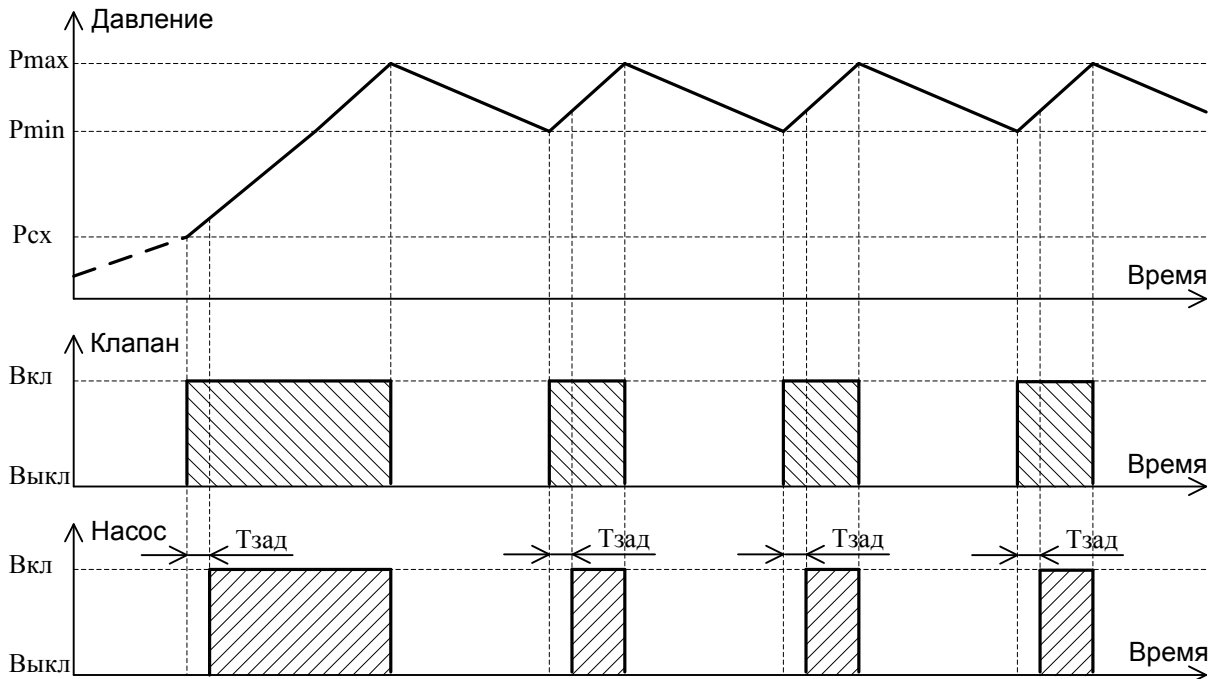
Рисунок 2 – Диаграмма работы по управлению подпиткой
