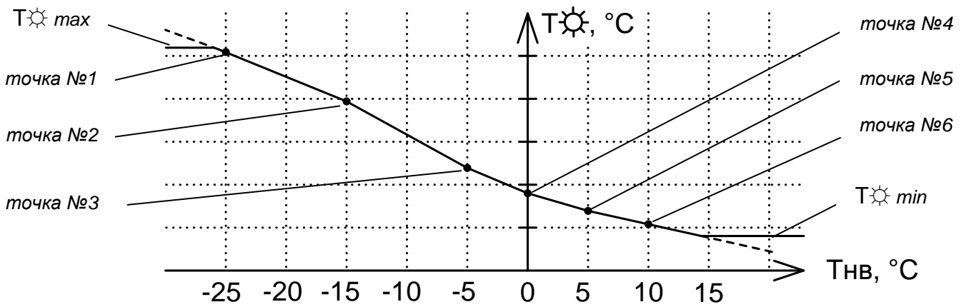
Рисунок 11 - Температурный график
